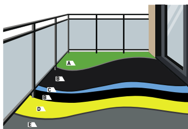
Tværsnit af gulvkonstruktionen
