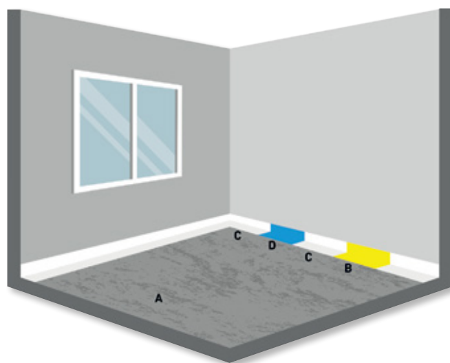
Poikkileikkaus sisäilmatiivistyksen ja radonsuojauksen rakenteesta
